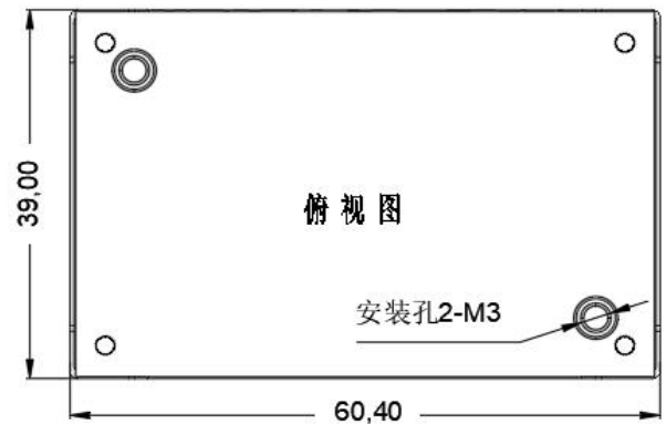
标准型 60.4*39.0*12.7mm
