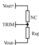
电压上调: 在Trim和输出负之间增加电阻Rup
